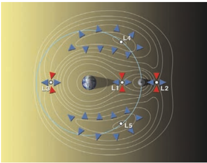
Lagrange Noktaları
